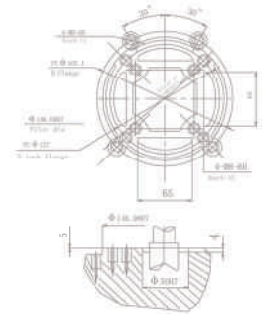
เพลารุ่น H186FAD
