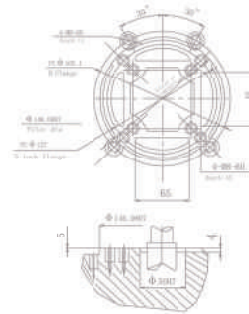
เพลารุ่น H186FD
