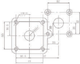
เพลารุ่น H170FD
